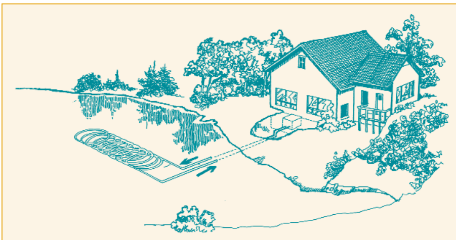
Les boucles de lac ou d'étang peuvent être utilisées aussi bien pour réchauffer que pour rafraîchir.
